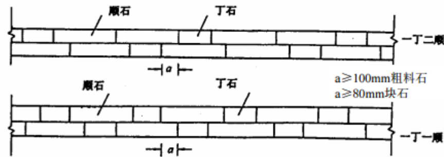
图413-5 镶面石砌筑
