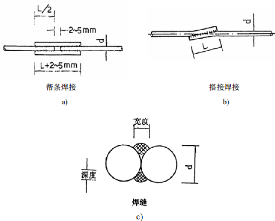
图403-1 电弧焊接
