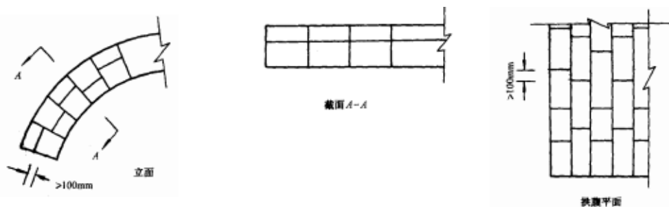
图413-6 相邻石块间搭接
